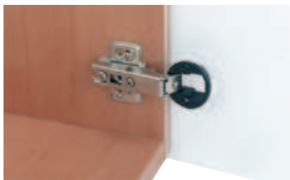
montaj în colț cu plăcuță de montaj
