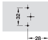
Schiță de găurire
