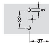
Schiță de găurire
