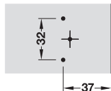
Schiță de găurire
