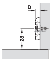
Schiță de găurire
