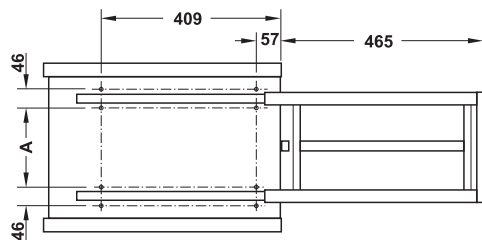
Auszugrahmen mit Fronthalter
